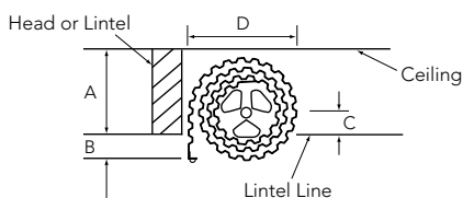
Door Roll Obtrusion Below Lintel
